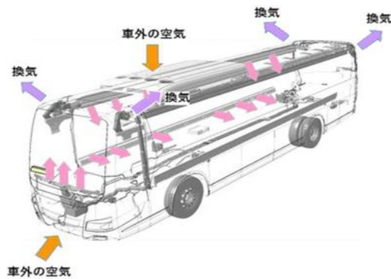
大型観光バス・天井A/Cタイプ
