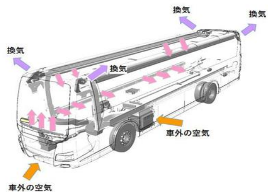
大型観光バス・床下A/Cタイプ
